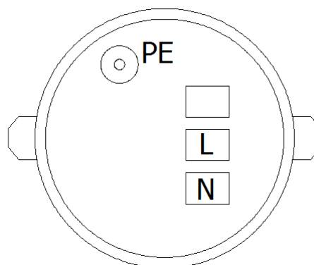
Рисунок 2 – Подключение
